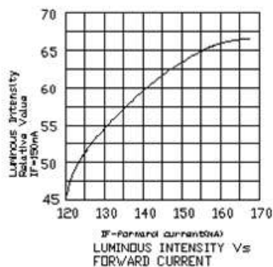
亮度与正向电流关系曲线图
