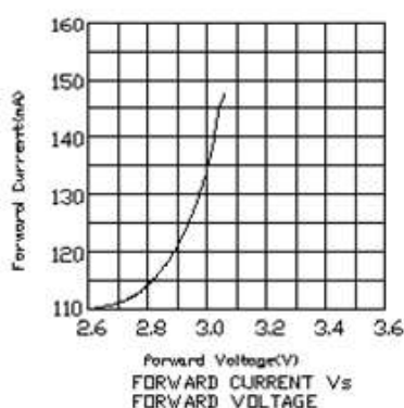
正向电流与正向电压关系曲线图
