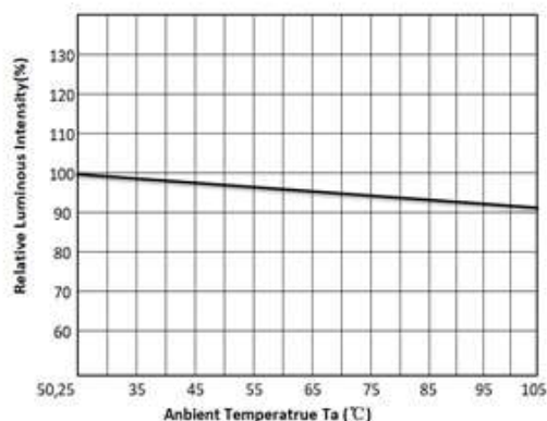
亮度与环境温度关系曲线图
