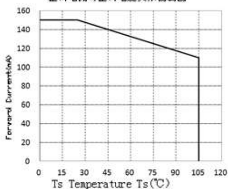
正向电流递减曲线图
