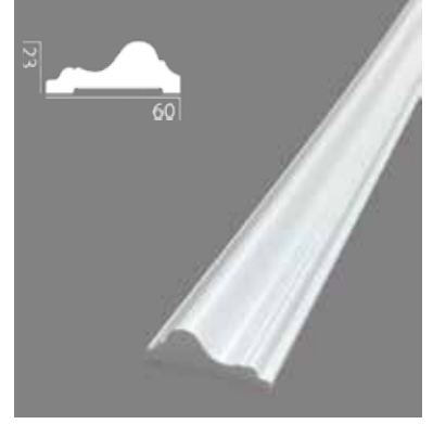
DB6017-D2 60x23x2400 mm
