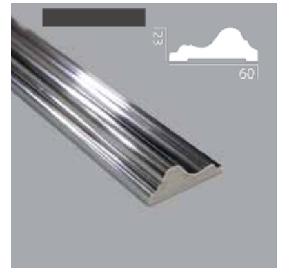
D6020-K 60x23x2400 mm
