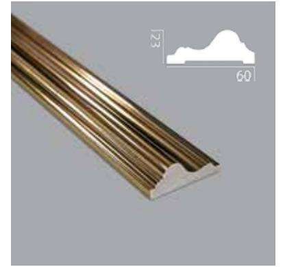
D6020-H 60x23x2400 mm
