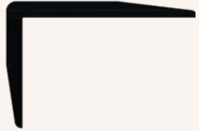
KAPLAMALI ( FOLYOLU ) L KÖŞE ( L EDGE CLOSURE )
