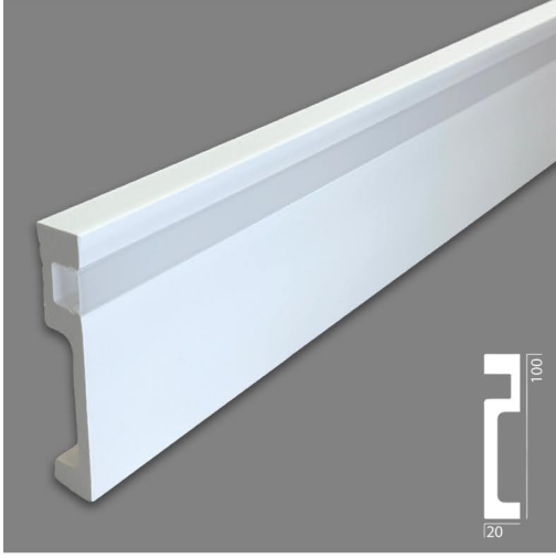
İSTANBUL LEDLİ SÜPÜRGELİK
