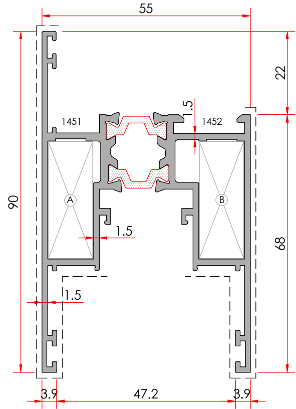
Kanat Profili
