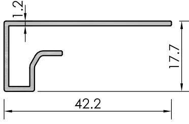
Dilatasyon Profili
