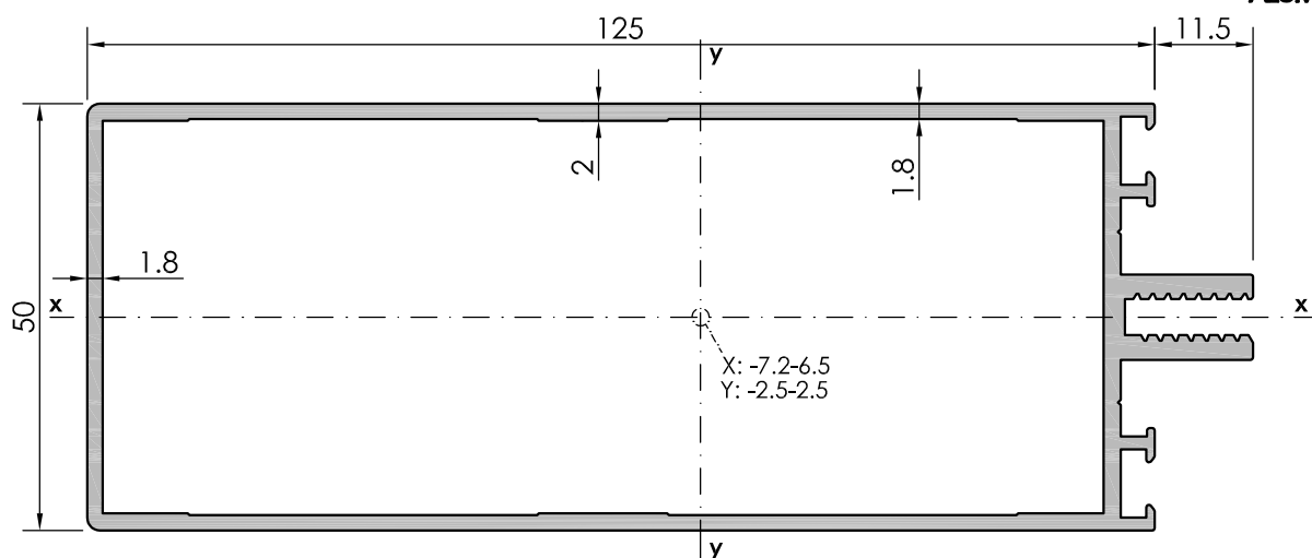
Transom
