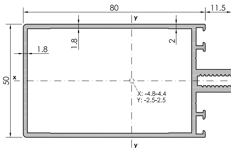
Transom
