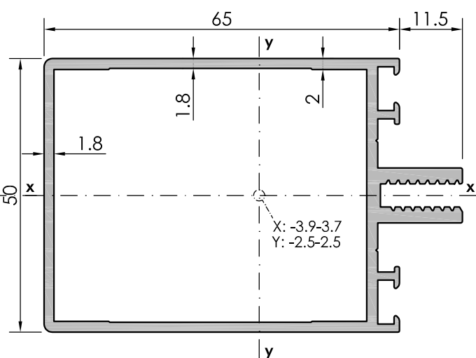
Transom
