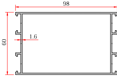
Meeting Rail - Orta Kayıt
