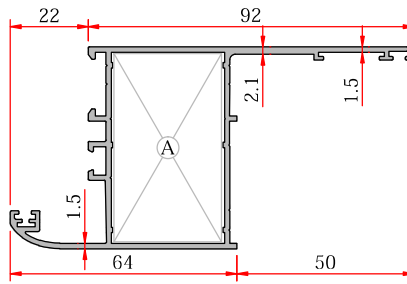
Sill Frame - Pervaz Kasa
