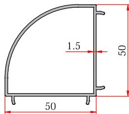
90° Corner Adapter 90° Köşe Dönüş Adaptörü
