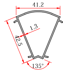
135° Corner Adapter 135° Köşe Dönüş Adaptörü
