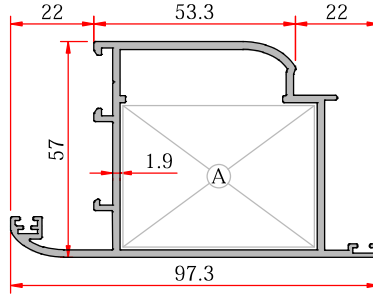
Outward Opening Vent - Dışa Açılır Kanat
