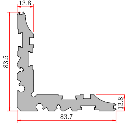
Corner Cleat - Kõşe Takozu
