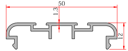
Swing Door Adapter Çarpma Kapı Adaptörü
