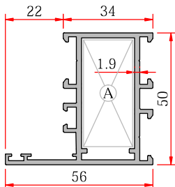
Wide Vent - Geniş Kasa
