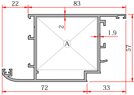
Door Vent - Kapı Kanat
