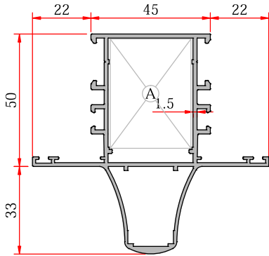
Reinforced Meeting Rail Takviyeli Orta Kayıt
