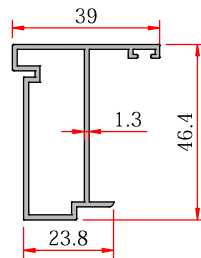
Outward Opening Middle Adapter Dışa Açılır Orta Adaptör
