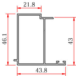
Outward Opening Adapter Dışa Açılır Adaptör
