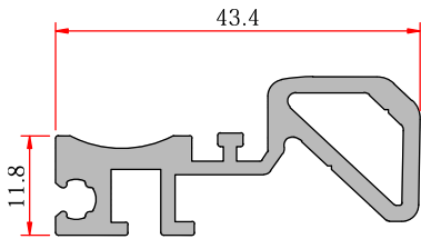
Meeting Rail Connection Orta Kayıt Baęlantı
