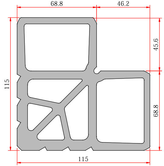
Corner Cleat - Kõşe Takozu
