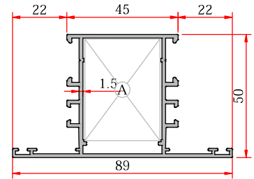
Meeting Rail - Orta Kayıt
