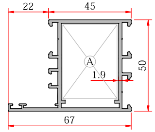
Wide Frame - Geniş Kasa
