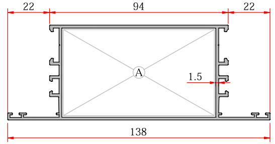
Base Meeting Rail - Baza Orta Kayıt
