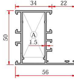
Wide Frame - Geniş Kasa
