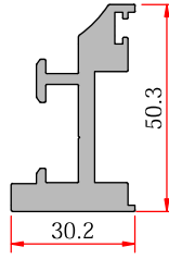
Pivoting Hinge - Pivot Menteşe
