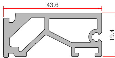
Meeting Rail Connection Orta Kayıt Baęlantı
