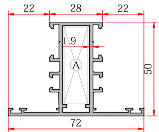
Narrow Meeting Rail - Dar Orta Kayıt
