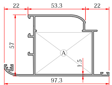
Outward Opening Vent - Dışa Açılır Kanat
