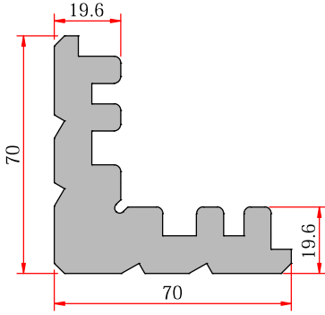
Corner Cleat - Kõşe Takozu
