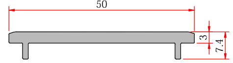
Swing Hinge Bottom - Çarpma Menteşe Altı
