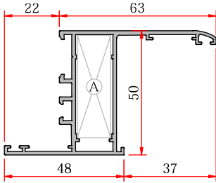
Sill Frame - Pervaz Kasa
