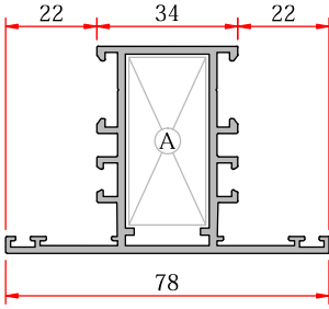
Meeting Rail - Orta Kayıt
