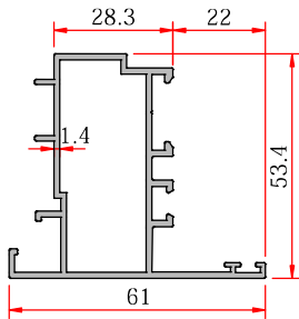
Double Vent Adapter - Çift Kanat Adaptörü
