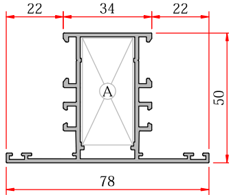
Meeting Rail - Orta Kayıt
