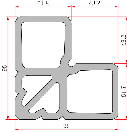
Corner Cleat - Kõşe Takozu
