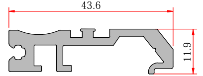
Meeting Rail Connection Orta Kayıt Baęlantı
