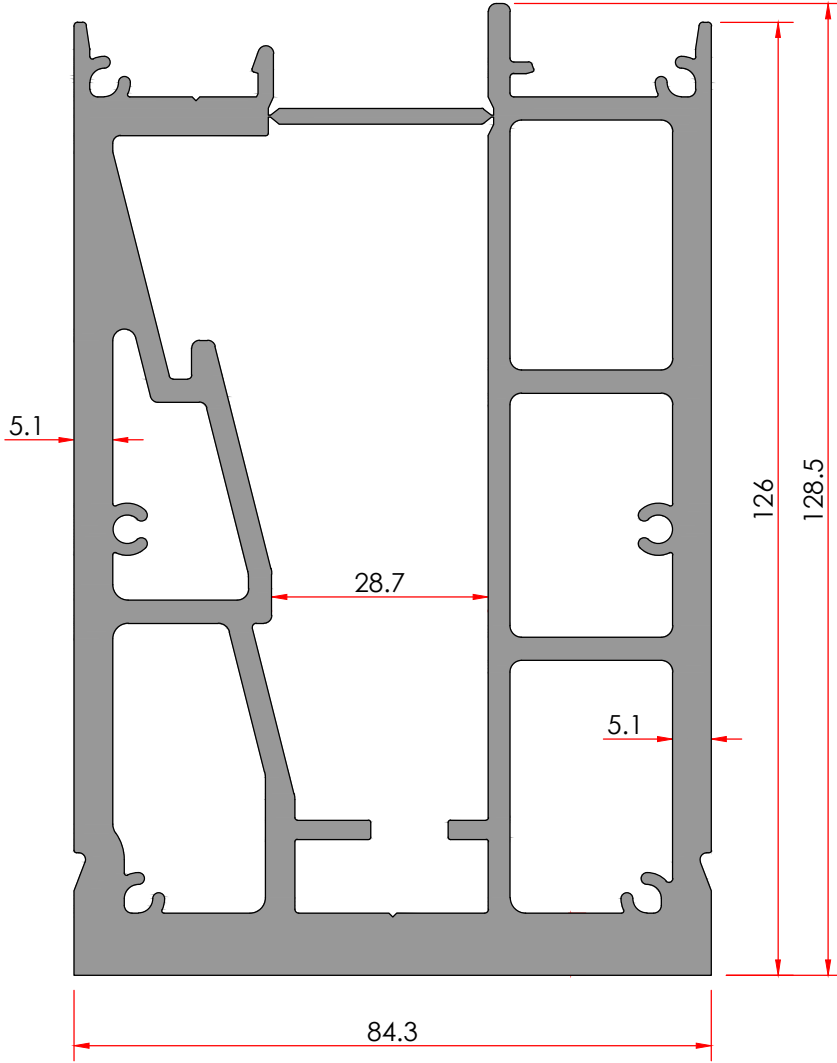
Küpeşte Ankrāj Profili
