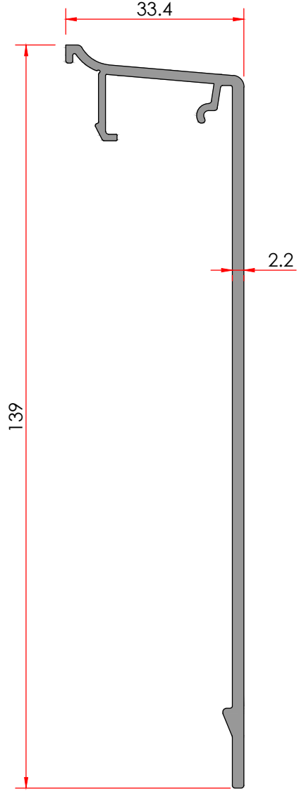
Küpeşte Kapak Profili
