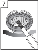
Üst değirmeni değirmen fırçası ile temizleyin
