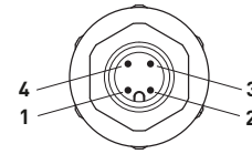
ERKEK KONNEKTÖR
