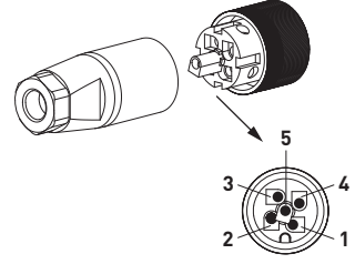
KABLO TARAFI
