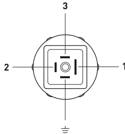
ERKEK KONNEKTÖR
