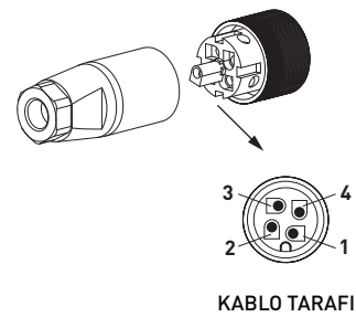
KABLO TARAFI
