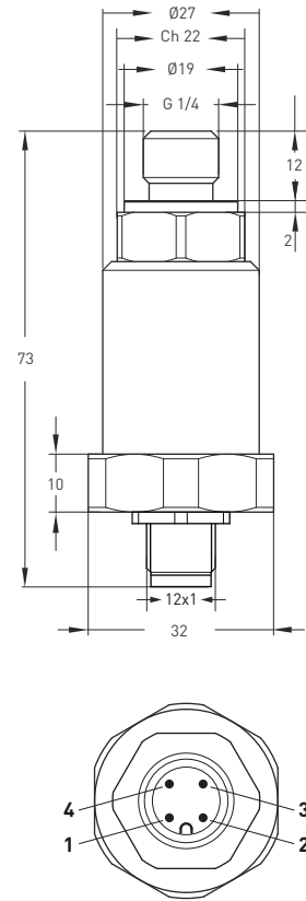
ERKEK KONNEKTÖR
