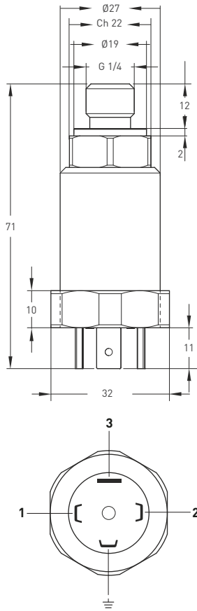
ERKEK KONNEKTÖR
