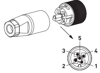
KABLO TARAFI
