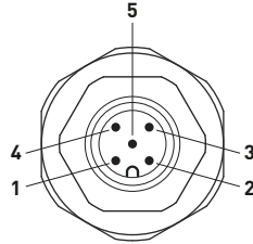
ERKEK KONNEKTÖR
