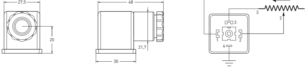
CN5A: 5 pin, M12 konnektör çıkışlı (opsiyonel)
