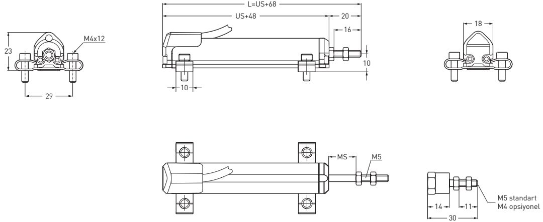
Kablo çıkışlı (standart)
