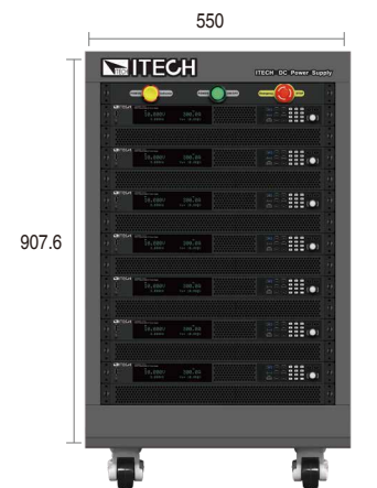
IT-E4029-15U (Dimension:mm)
