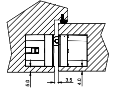
Hinge Application / Menteşe uygulama ölçüsü
