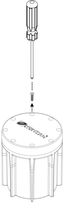
Şekil 10 - Tornavida yardımı ile vidanın(1) sökülmesi
