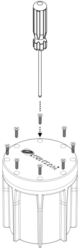
Şekil 12 - Tornavida yardımı ile üst kapağın kapatılması
