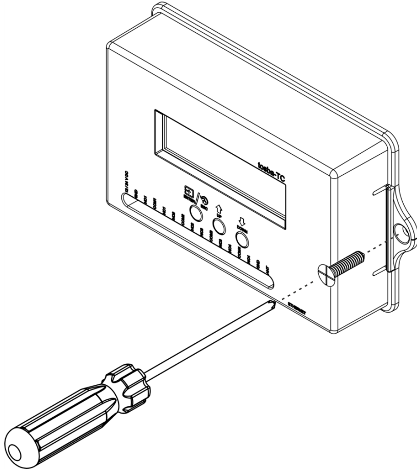
Şekil 16 - Bir tornavida yardımı ile ilgili bölgeye sabitleyiniz.
