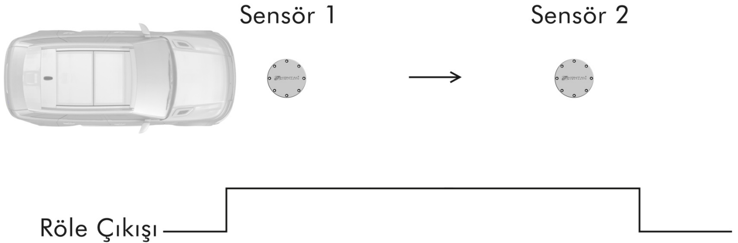
Şekil 3 - Seri Mod
