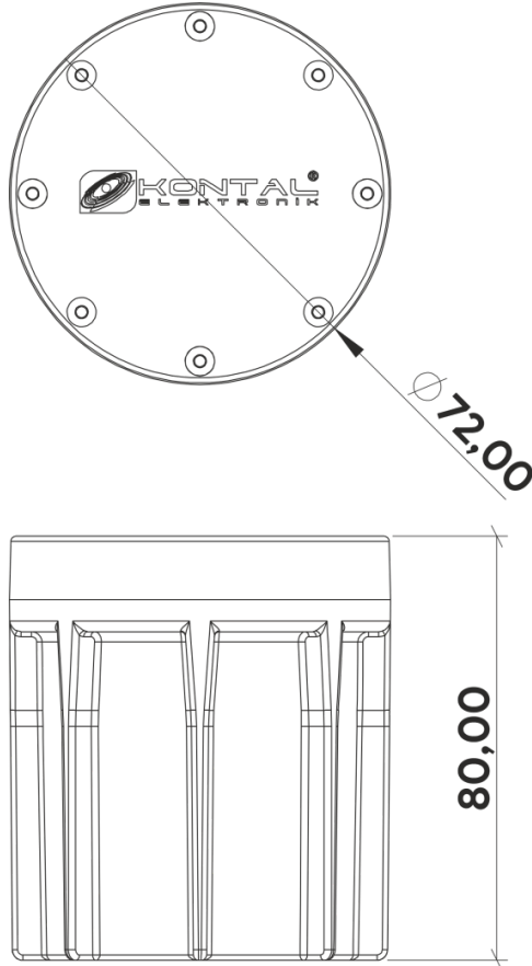
Şekil 15- Boyutlar(mm)
