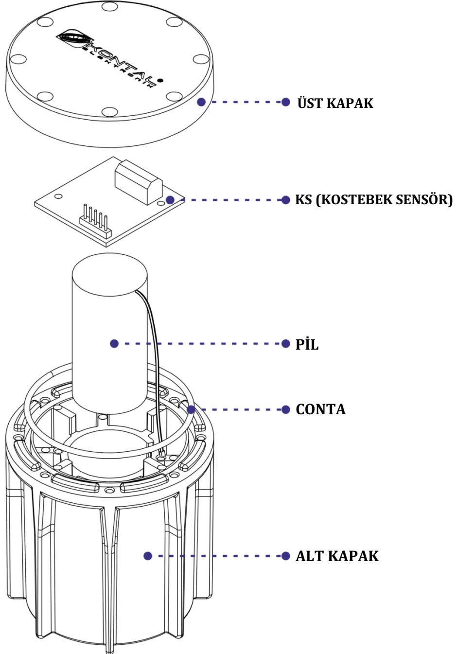
Şekil 9 - KS kartı iç yapısı
