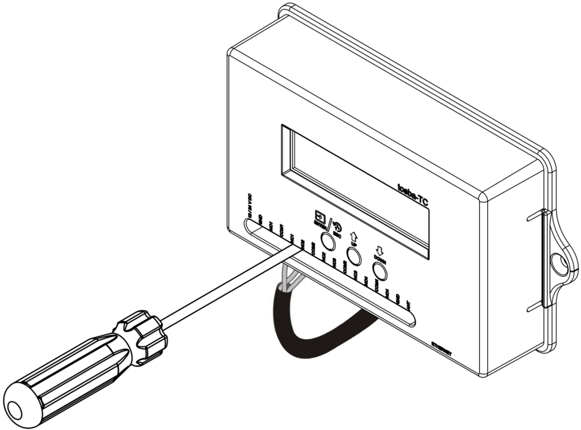
Şekil 17 - Klemens bağlantılarınızı yapınız.
