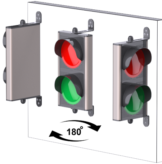
Şekil 8-TRFL Açı Ayarlama
