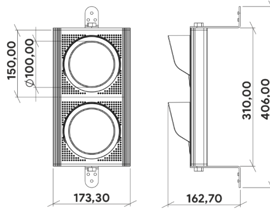
Şekil 4-TRFL1 Ölçüler
