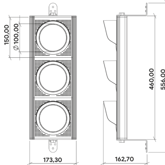
Şekil 5-TRFL2 Ölçüler
