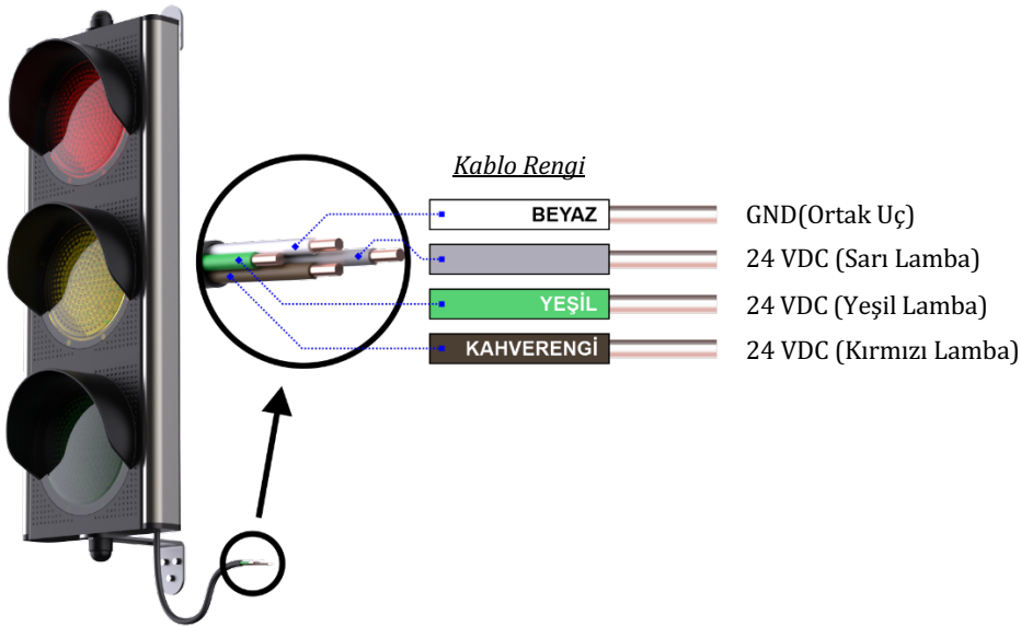
Şekil 3 - TRFL3 Kablo Bağlantı Şeması
