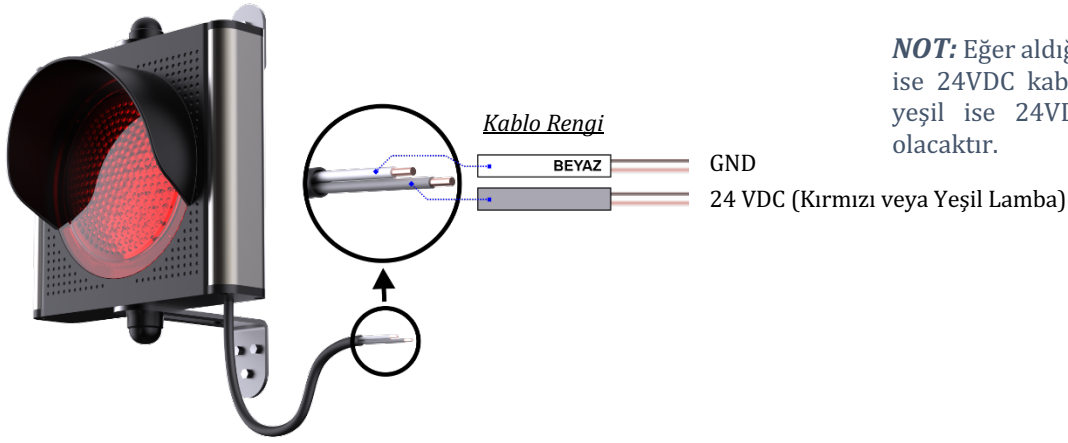
Şekil 1-TRFL1 Kablo Bağlantı Şeması
