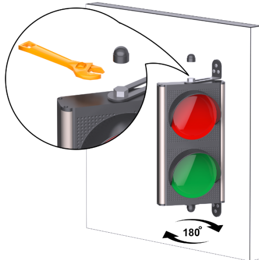
Şekil 9-TRFL Sabitleme ve Somun Kapaklarının Kapanması
