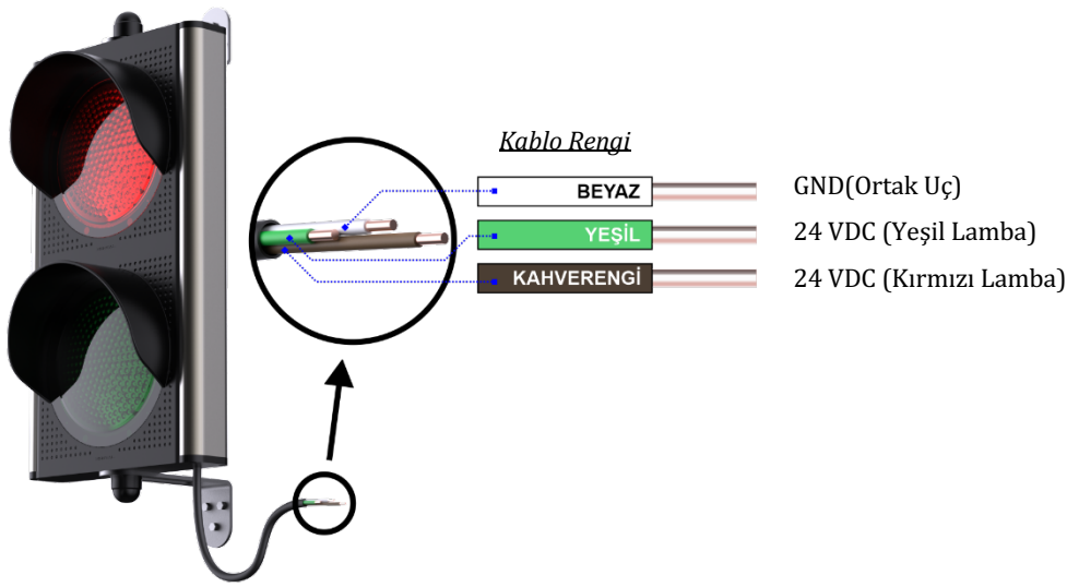
Şekil 2 - TRFL2 Kablo Bağlantı Şeması
