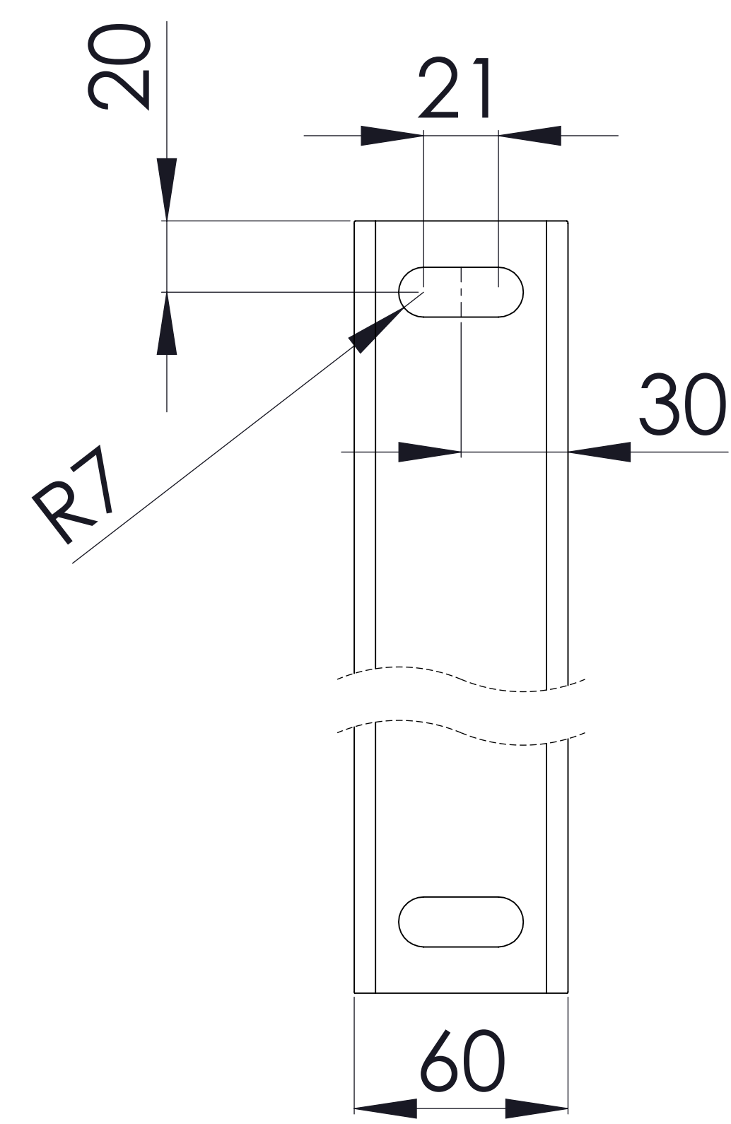
KESİT A-A ÖLÇEK 1 : 1.5
