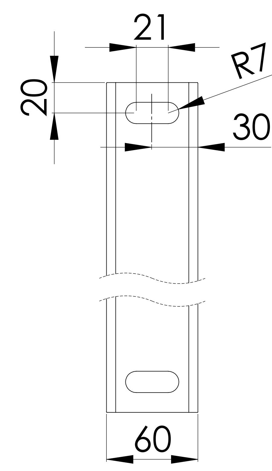
KESİT A-A ÖLÇEK 1 : 1.5
