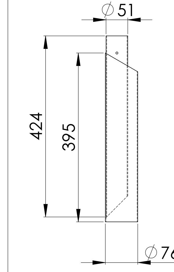
ÇIKIŞ BORUSU DETAY
