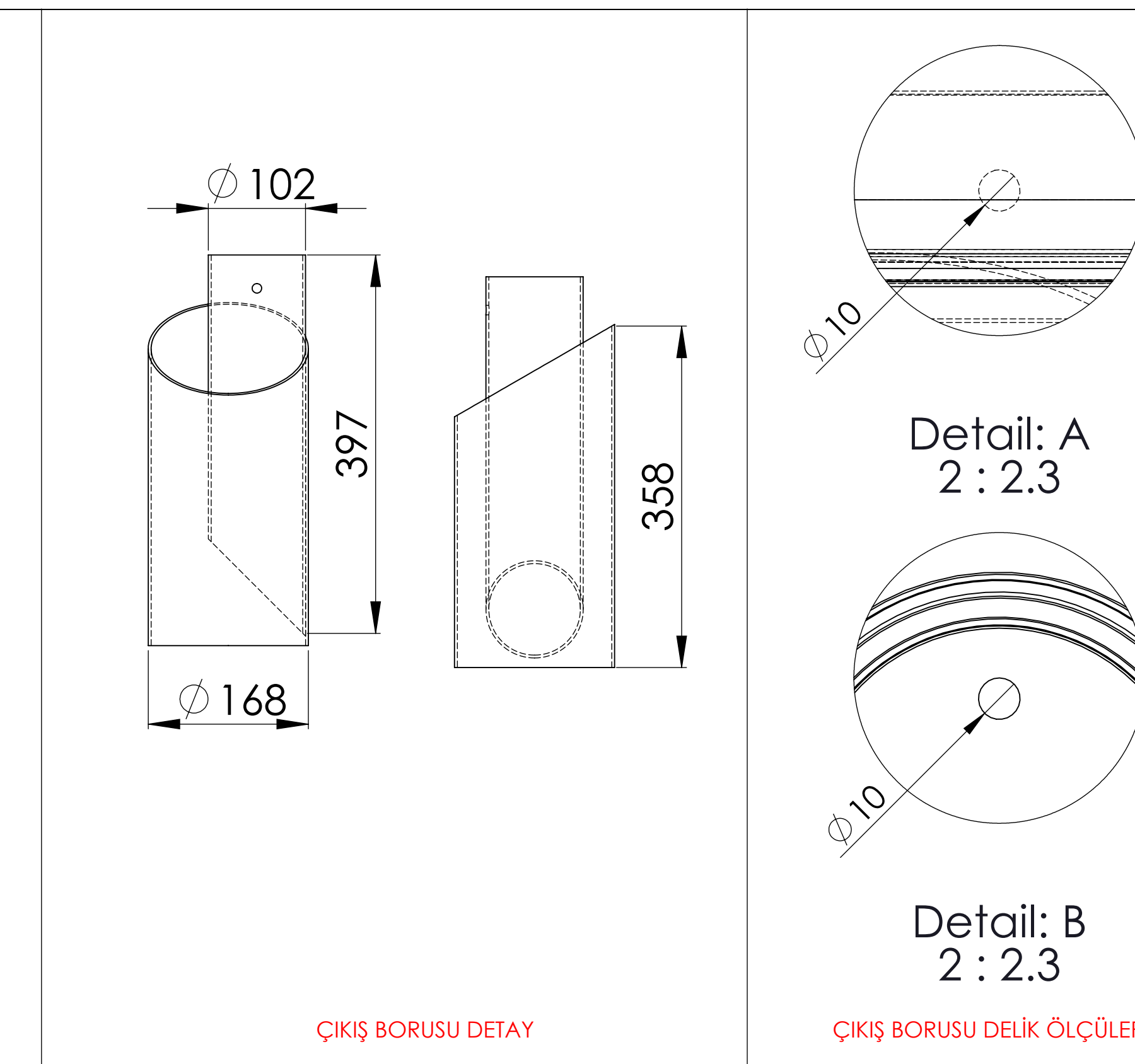
ÇIKIŞ BORUSU DETAY
