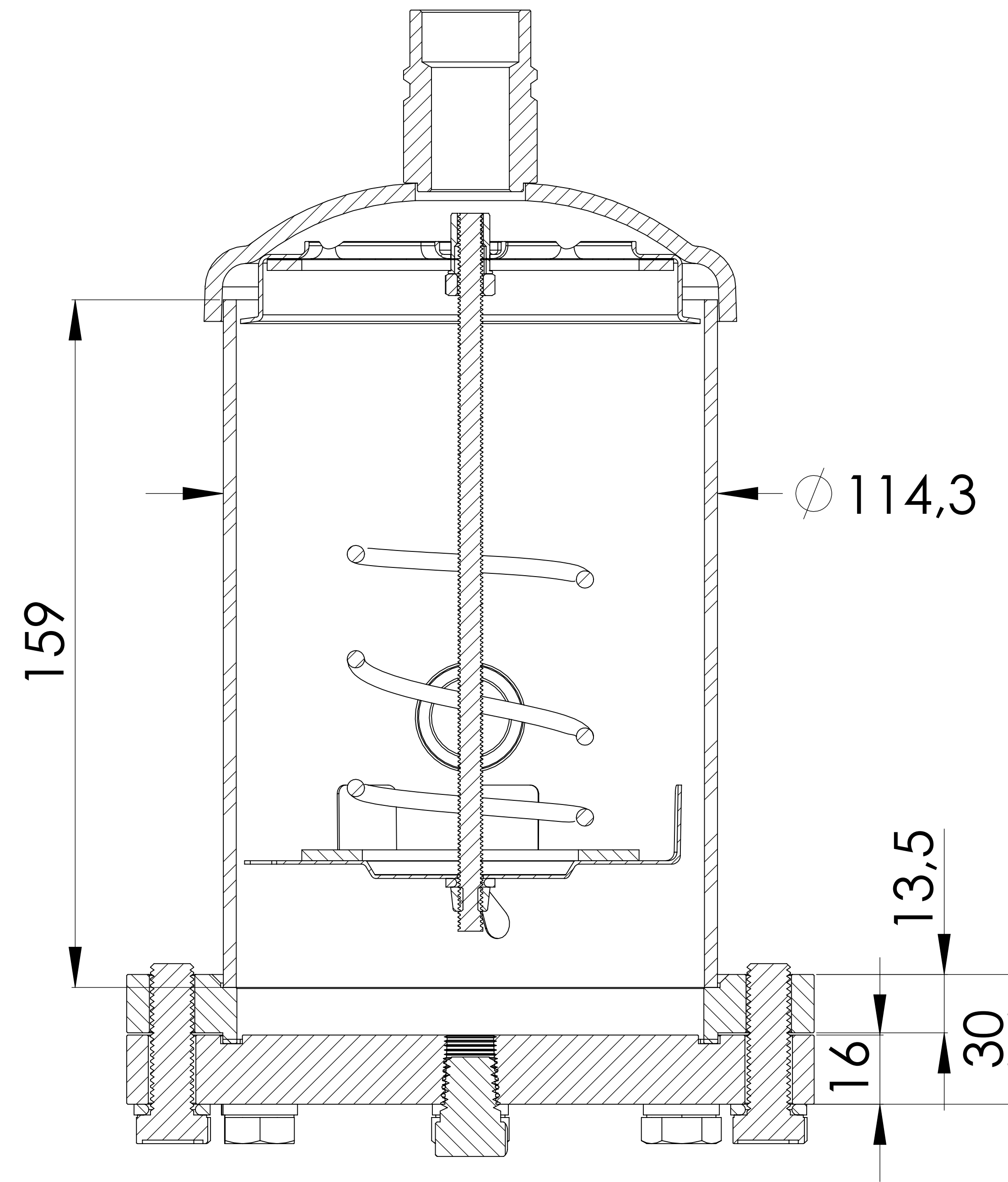
KESIT A-A ÖLÇEK 1:0,8
