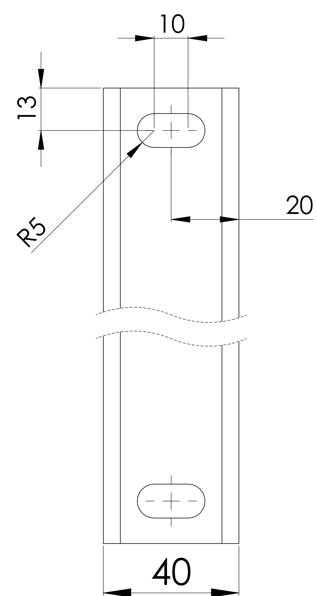
KESİT A-A ÖLÇEK 1 : 0.7
