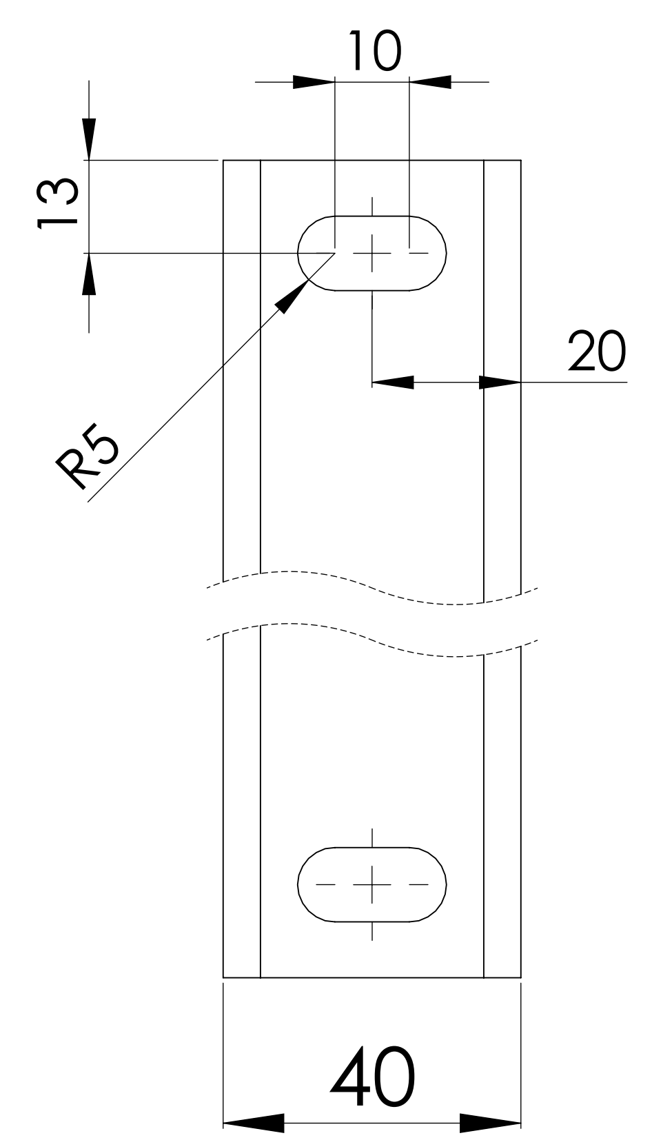
KESIT A-A ÖLÇEK 1 : 0.7
