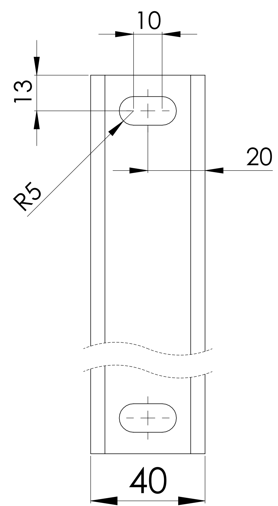
KESIT A-A ÖLÇEK 1 : 0.8
