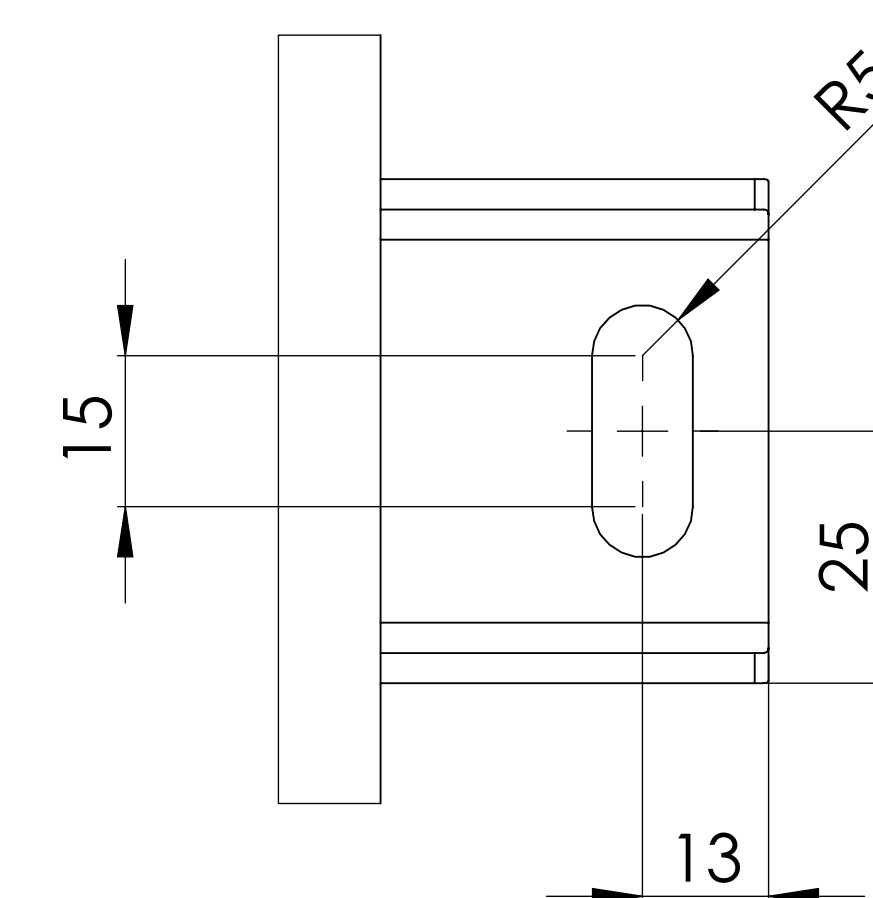
Detail: A 2 : 1.5
