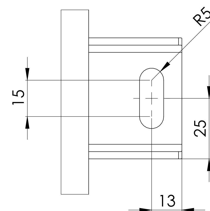
Detail: A 2 : 1.5
