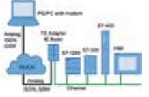
Teleservis Adaptörü
