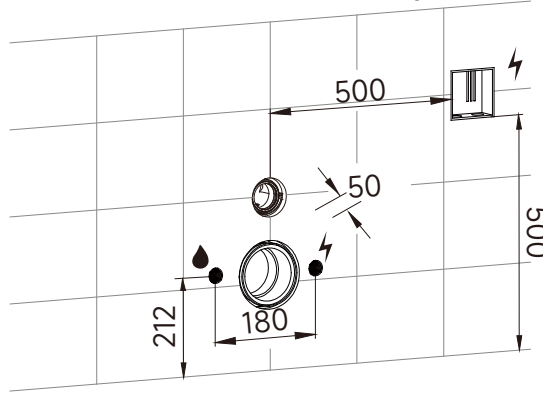
Su ve Elektrik ön kurulum ölçüleri
