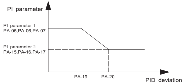
Figür 6-25 PID parametresi anahtarlama diagramı
