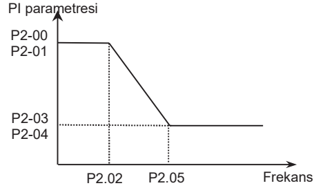
Figure 6-2 PI parametre diagramı
