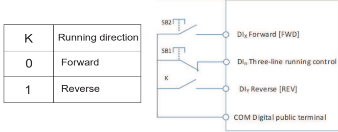
Figure 6-8 Üç Kablolu Çalışma Modu 2
