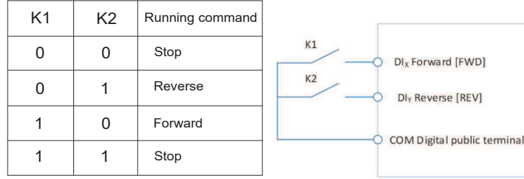
Şekil 6-5 İki Kablolu Çalışma Modu 1
