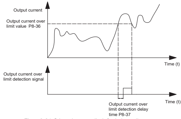
Figür 6-21 Çıkış akımı üst limit fonksiyon diyagramı
