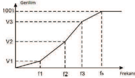
Figure 6-4 V/F Eğrisi ayar diagramı
