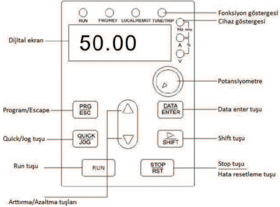
Figür 4-1 Tuş Takımı Diagramı
