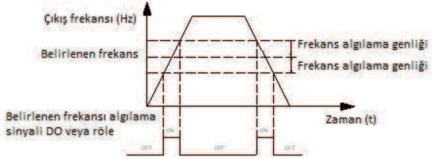
Figür 6-19 Belirlenen frekans algılama diyagramı
