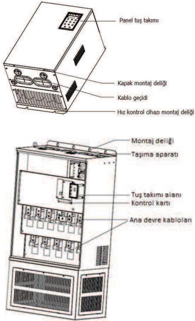
Figür 2-3 Hız kontrol cihazı parçaları
