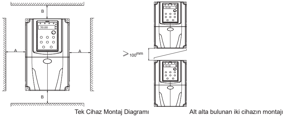
Figür 3-1 Montaj Diagramı
