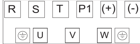
Figür 3-10 Bağlantı diagramı (3 faz 380V, 90~710 kW)
