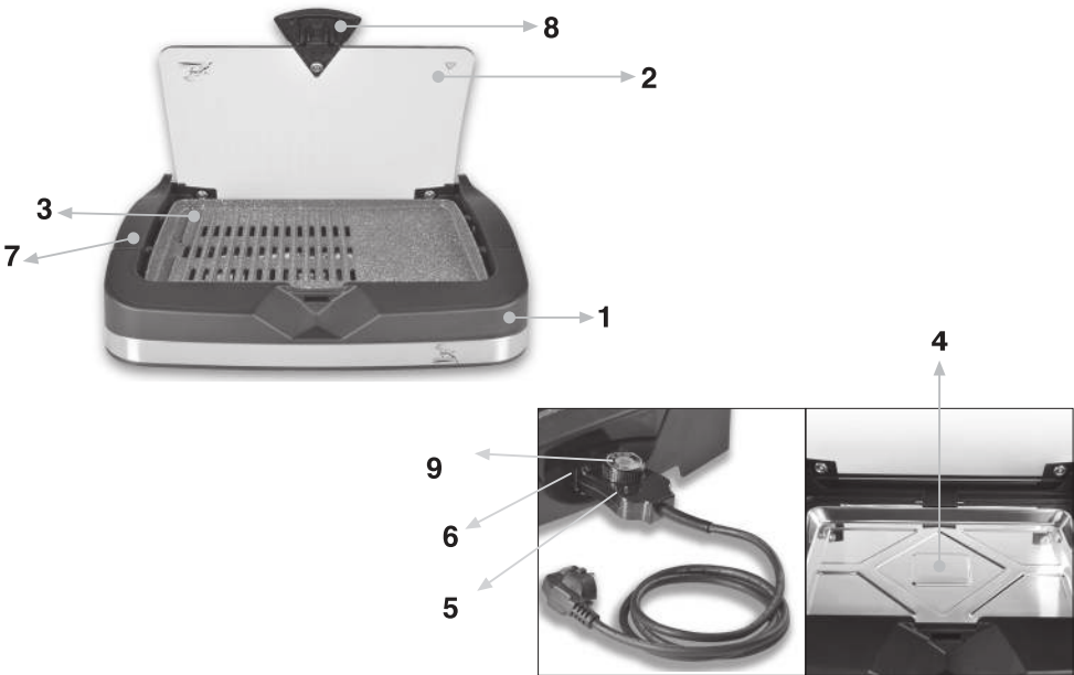
(1) Hauptkörper (2) Deckel aus Glas (3) Grillrost (4) Fettauffangschale (5) Thermostat (6) Thermostatanschluss (7) Griff (8) Deckelverriegelung und Griff (9) Temperaturregelung
