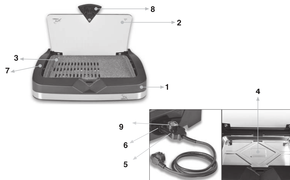
(1) Partie principale (2) Couvercle en verre (3) Barbecue (4) Bac à graisse (5) Thermostat (6) Raccordement thermostat (7) Poignée (8) Couvercle verrouillable et poignée (9) Réglage de température
