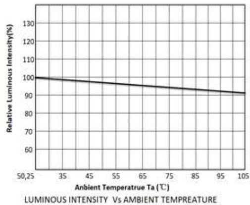
亮度与环境温度关系曲线图
