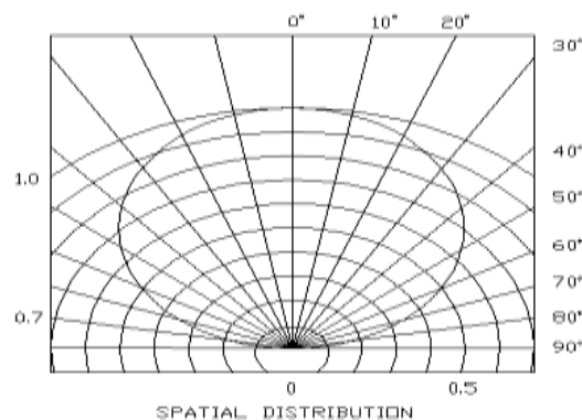
发光角度图解
