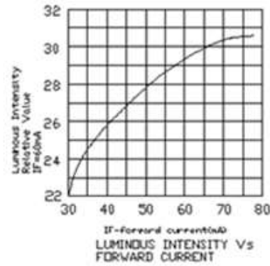
亮度与正向电流关系曲线图
