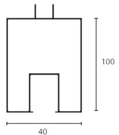
100 Lük Kablo kanalı
