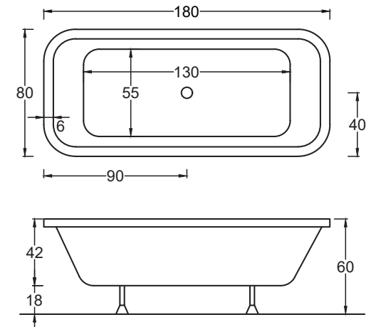
ESSENCE/DIONE TEKNİK ÇİZİM:
