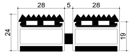
KESİT DETAYI
