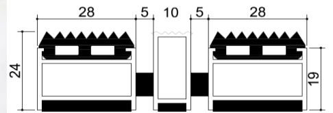
KESİT DETAYI
