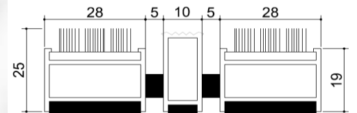
KESİT DETAYI
